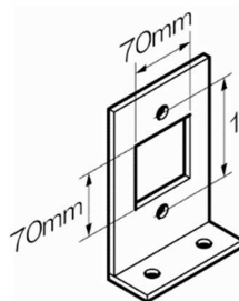
ブラケット
